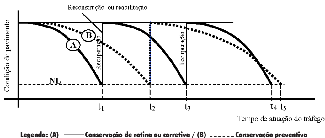
FIGURA 2 – ANÁLISE DA POSTERGAÇÃO DAS INTERVENÇÕES NOS PAVIMENTOS
